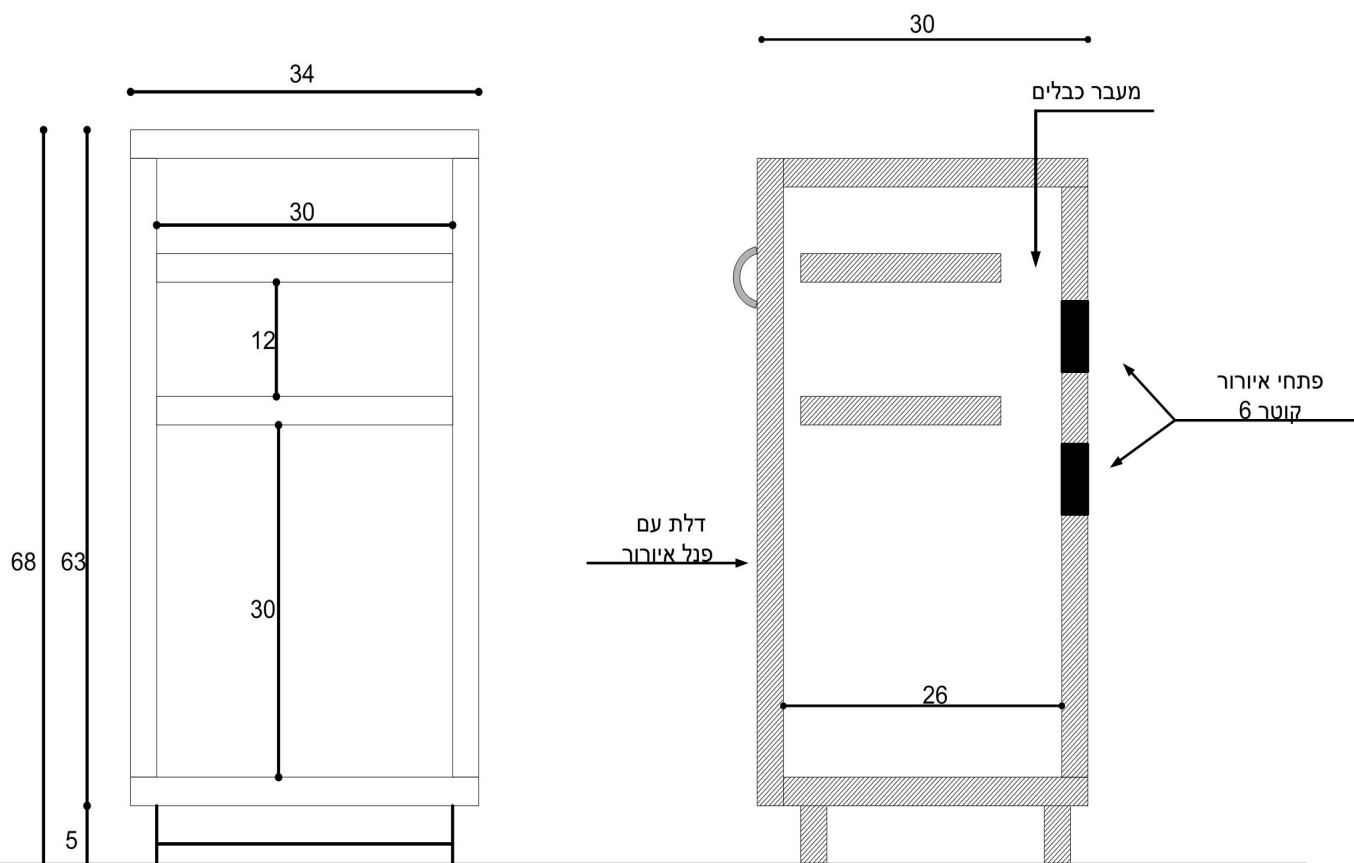
חזית ( ללא הדלת)
